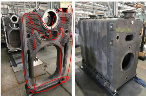
図 23 セクション（ウェットボトム形）の外観
