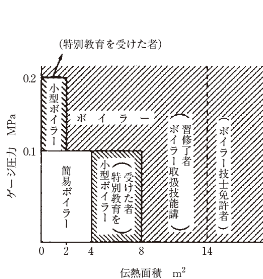
(b-1) 温水ボイラー（木質バイオマス温水ボイラー以外）
