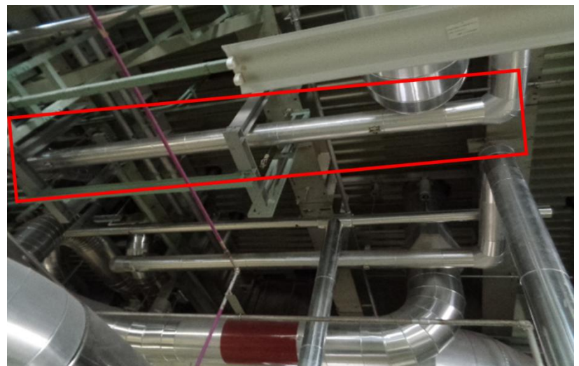
図 2.52 保温材（発電）
