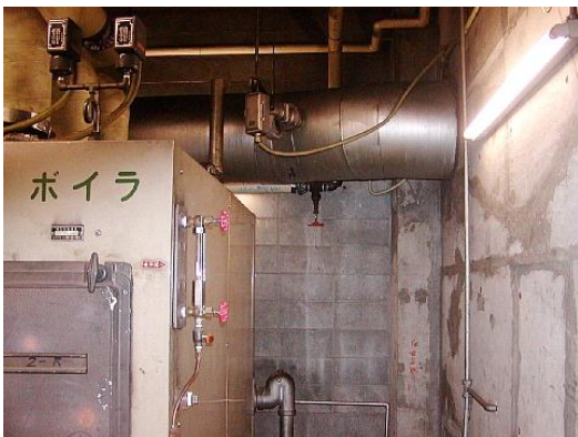
B1Fボイラー室。正面は横引き煙道(断熱材未確認)。左から右にRC部に挿入
